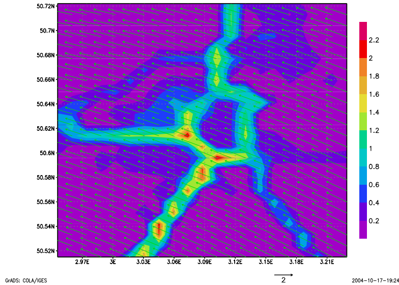
FIG. 5.1 – Emissions surfaciques moyennes de NO en \mu\text{gm}^{-2}\text{s}^{-1} et vent moyen au sol en \text{m.s}^{-1} pour le 11 Mai.
