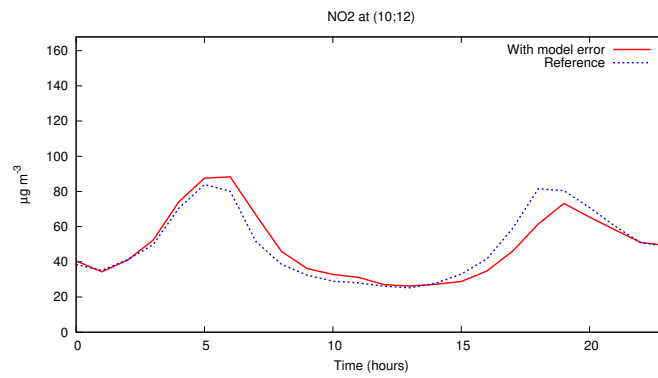
FIG. 5.20 – Concentrations de \text{NO}_2 à une station de Lille le 11 Mai. Valeurs de référence et valeurs avec une erreur modèle.
