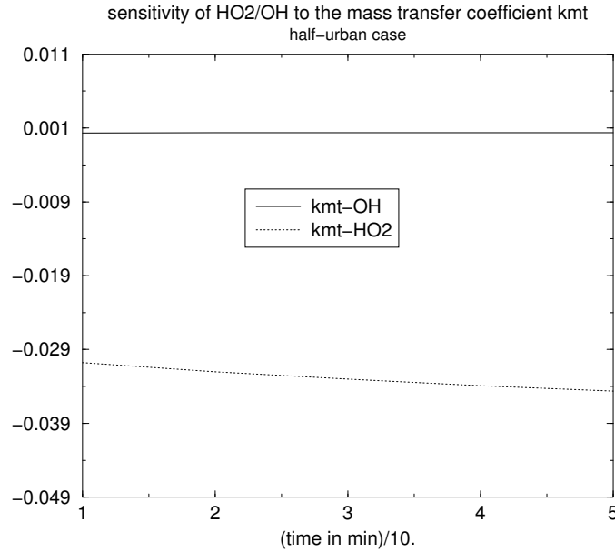
FIG. 4.2 – Sensibilité du ratio \frac{\text{HO}_2}{\text{OH}} au coefficient de transfert de masse k_{mt} .
