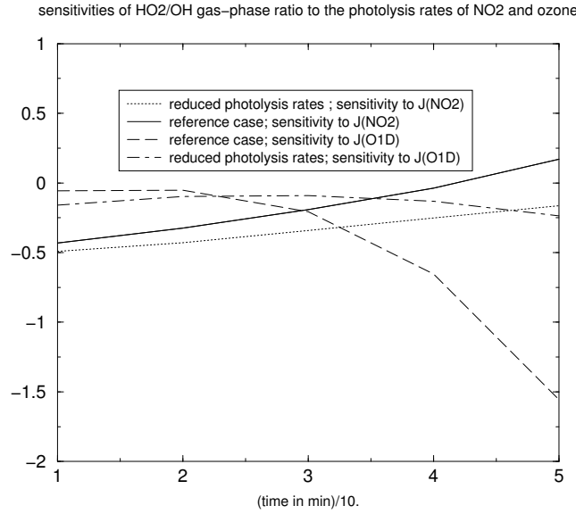
FIG. 4.3 – Sensibilité du ratio \frac{\text{HO}_2}{\text{OH}} aux taux de photolyse de \text{NO}_2 et \text{O}_3 .
