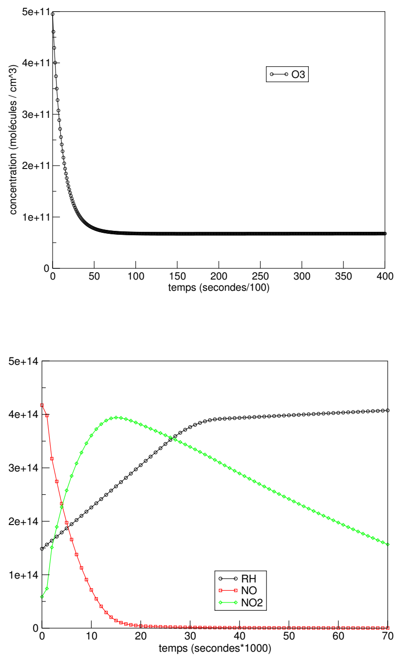
FIG. B.3 – Evolution temporelle des concentrations de NO, NO 2 et RH.
