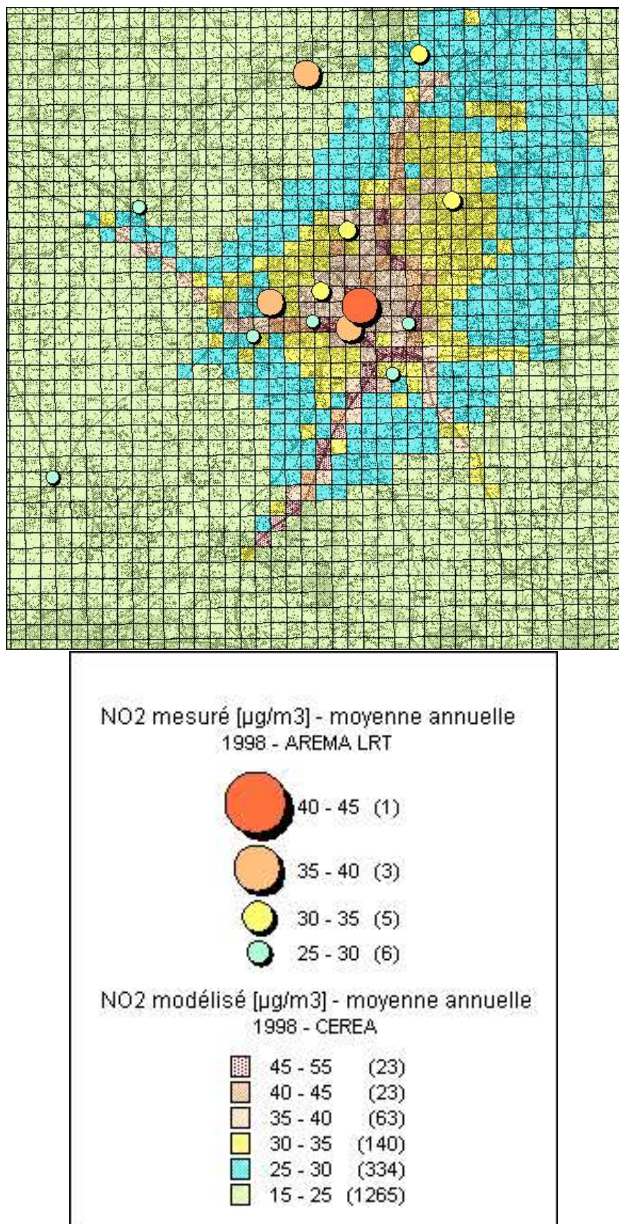
FIG. 2.10 – Moyenne annuelle du dioxyde d'azote.
