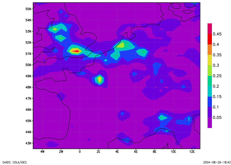
FIG. 1.10 – Emissions surfaciques moyennes de \text{NO}_x ( \mu\text{g.m}^{-2}\text{s}^{-1} ).
