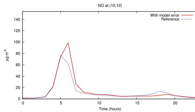
FIG. 5.21 – Concentrations de \text{NO} à une station de Lille le 11 Mai. Valeurs de référence et valeurs avec une erreur modèle.
