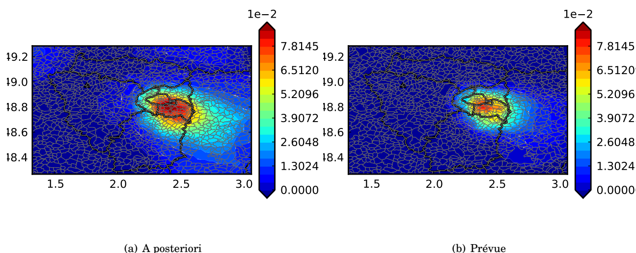
FIGURE 5.55 – Champs de probabilité a posteriori et prévu pour l'évènement [\text{NO}_2] \geq 100 \mu\text{gm}^{-3} , à la date du 27 janvier 2007 dans la région Île-de-France.
