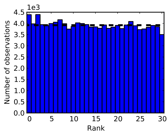
(b) Diagramme de rang calibré avec B
