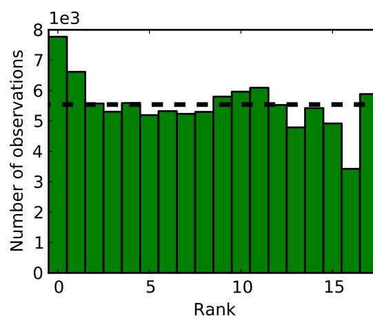
(b) Diagramme de rang calibré sur A
