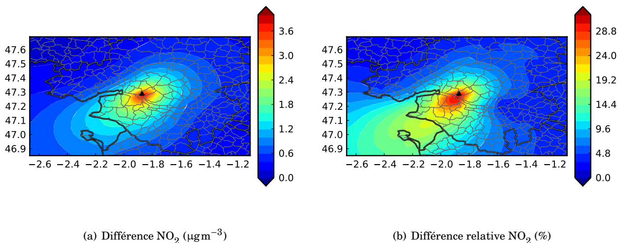
FIGURE 5.28 – Impact moyen absolu ( \mu\text{gm}^{-3} ) et relatif (%) du champ de \text{NO}_2 dans la région des Pays de la Loire.
