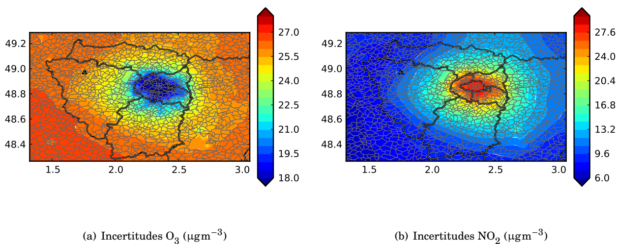
FIGURE 5.8 – Cartes d'incertitudes moyennes pour O_3 et NO_2 en \mu\text{gm}^{-3} pour le domaine Île-de-France issues des sous-ensembles calibrés via le diagramme de rang.
