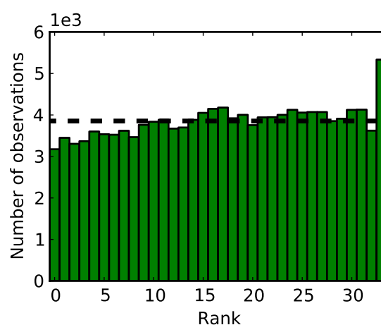
(b) Diagramme de rang calibré avec A
