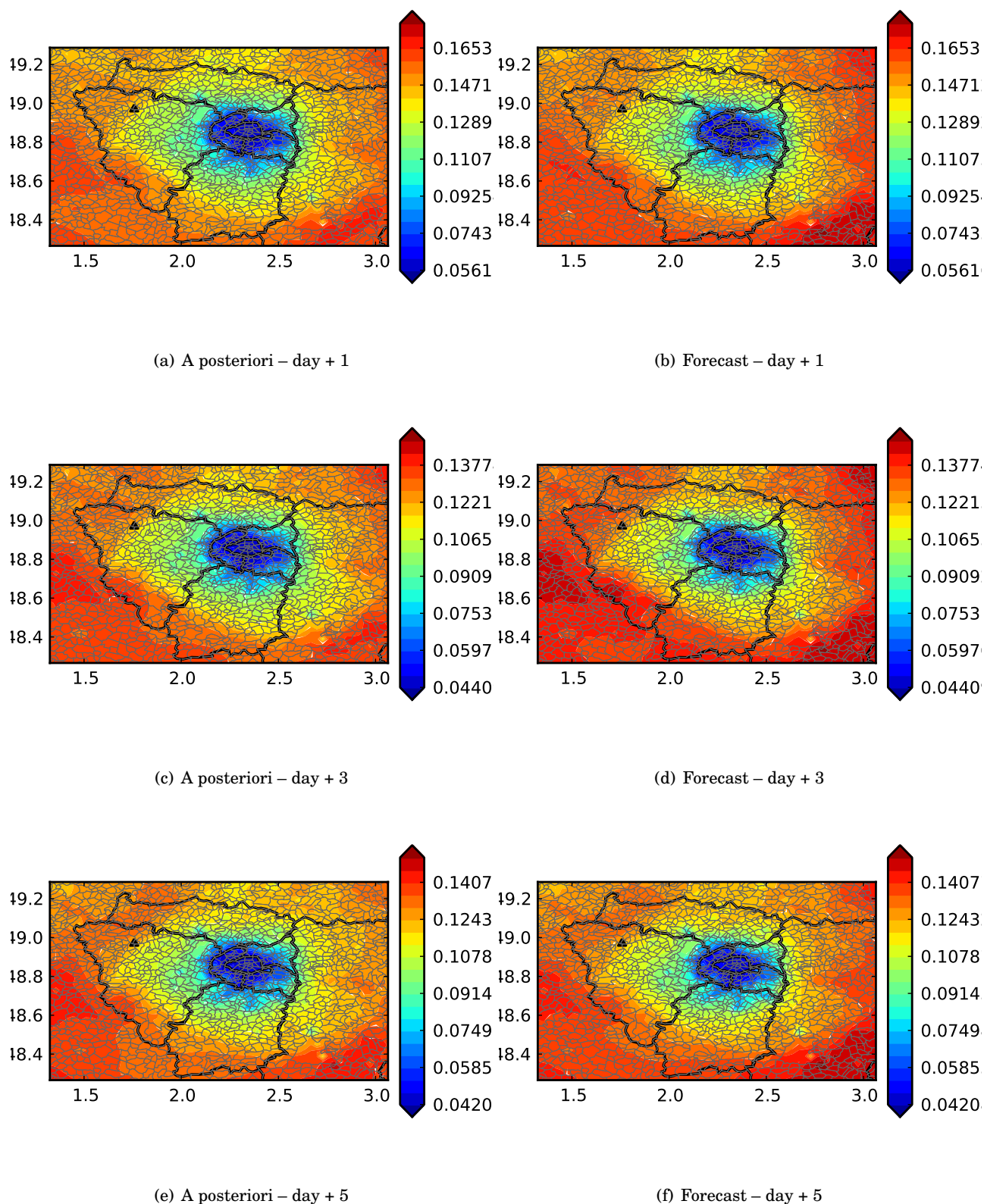
FIGURE 5.52 – Champs de probabilité a posteriori et prévu d'occurrence de l'évènement [O_3] \geq 80 \mu\text{gm}^{-3} , moyennés sur toute la période, pour les 1 er , 3 e et 5 e jours suivants les périodes d'apprentissage dans la région Île-de-France.
