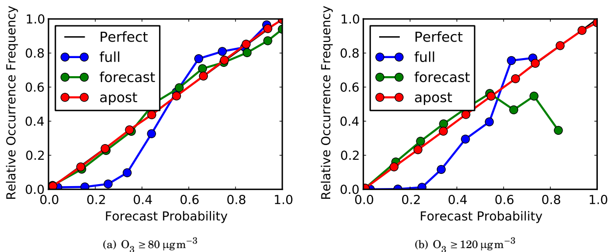
FIGURE 5.50 – Diagrammes de fiabilité cumulés issus de plusieurs prévisions pour les deux évènements [O_3] \geq 80 \mu\text{gm}^{-3} et \geq 120 \mu\text{gm}^{-3} dans la région de Porcheville. La courbe verte correspond au diagramme de fiabilité issu des sous-ensembles calibrés prévus, en rouge au diagramme issu des sous-ensembles calibrés a posteriori et en bleu, celui de l'ensemble complet.
