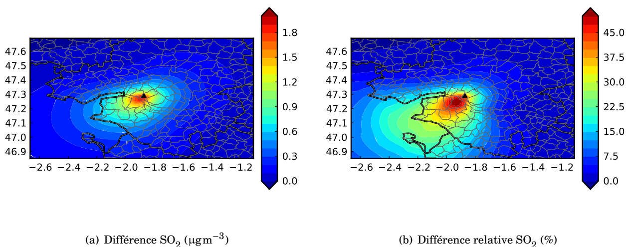
FIGURE 5.29 – Impact moyen absolu ( \mu\text{gm}^{-3} ) et relatif (%) du champ de \text{SO}_2 dans la région des Pays de la Loire.
