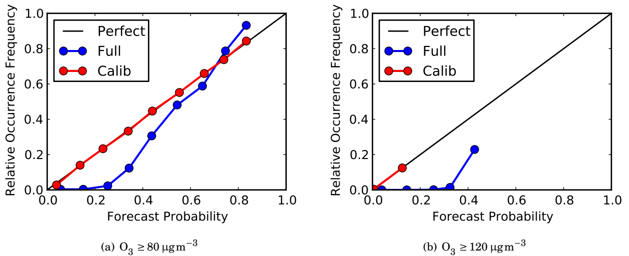
FIGURE 5.21 – Diagrammes de fiabilité de l'ensemble complet et du sous-ensemble calibré de l'ozone de la région de Cordemais pour les événements [O_3] \geq 80 \mu\text{gm}^{-3} et \geq 120 \mu\text{gm}^{-3} .
