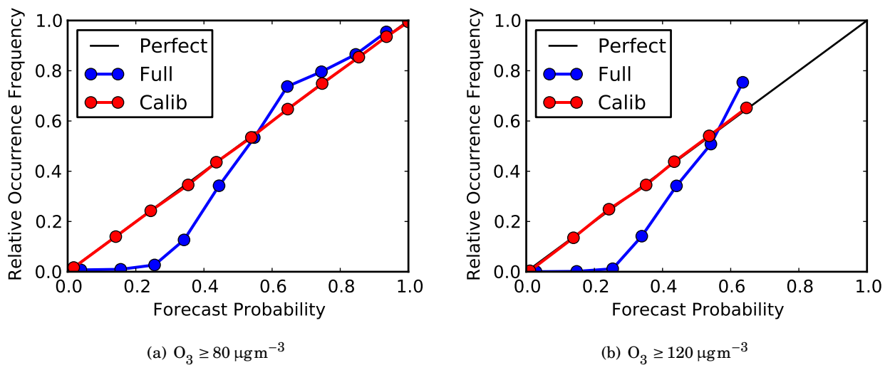
FIGURE 5.17 – Diagrammes de fiabilité de l'ensemble complet et du sous-ensemble calibré d'ozone de la région de Porcheville pour les évènements [\text{O}_3] \geq 80 \mu\text{gm}^{-3} et \geq 120 \mu\text{gm}^{-3} .
