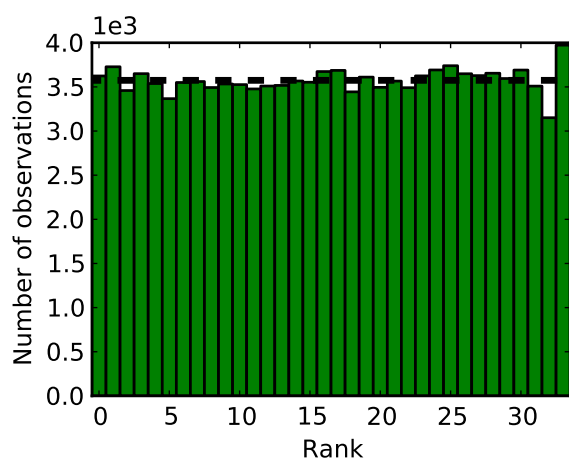
(a) Diagramme de rang calibré avec A
