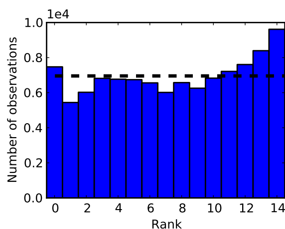
(b) Diagramme de rang calibré sur B
