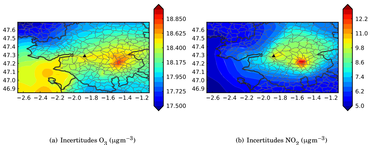
FIGURE 5.14 – Cartes d'incertitude moyenne de \text{O}_3 et \text{NO}_2 en \mu\text{gm}^{-3} pour le domaine Pays de la Loire issues des sous-ensembles calibrés via le diagramme de rang.
