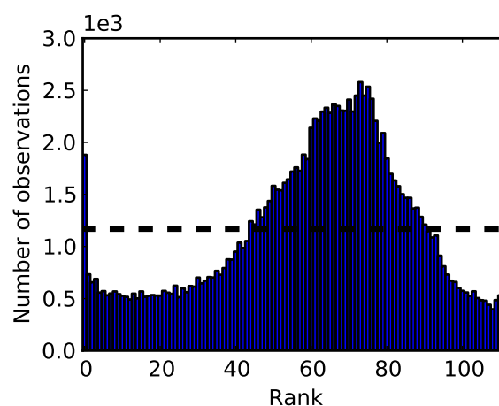
(b) Diagramme de rang complet sur B
