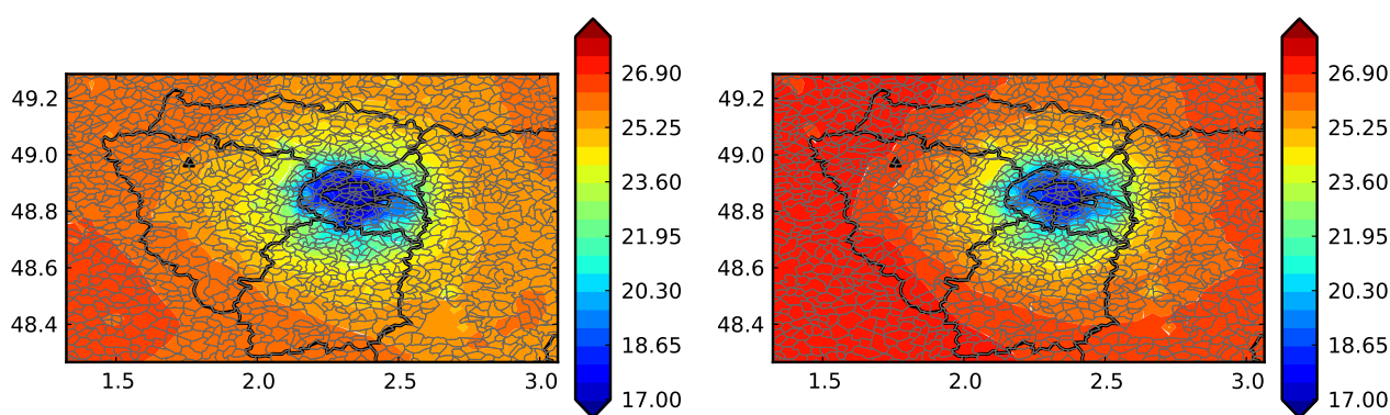
(a) Incertitude O_3 ( \mu\text{gm}^{-3} ) issue de la calibration avec le réseau A
