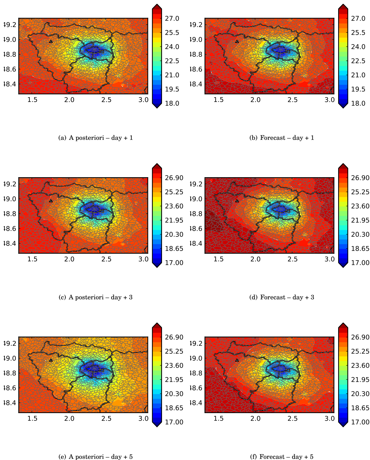
FIGURE 5.46 – Champs d'incertitude d'ozone a posteriori et pr vu moyenn s sur toute la p riode, pour les 1 er , 3 e et 5 e jours suivants les p riodes d'apprentissage dans la r gion  le-de-France (en \mu\text{g m}^{-3} ).
